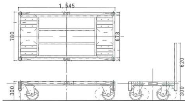
ハコボーダイFC-3型
